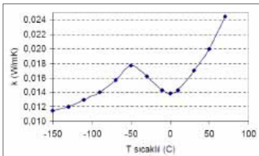
Sıcaklığın PUR ısı iletkenliği üzerindeki etkisi.
