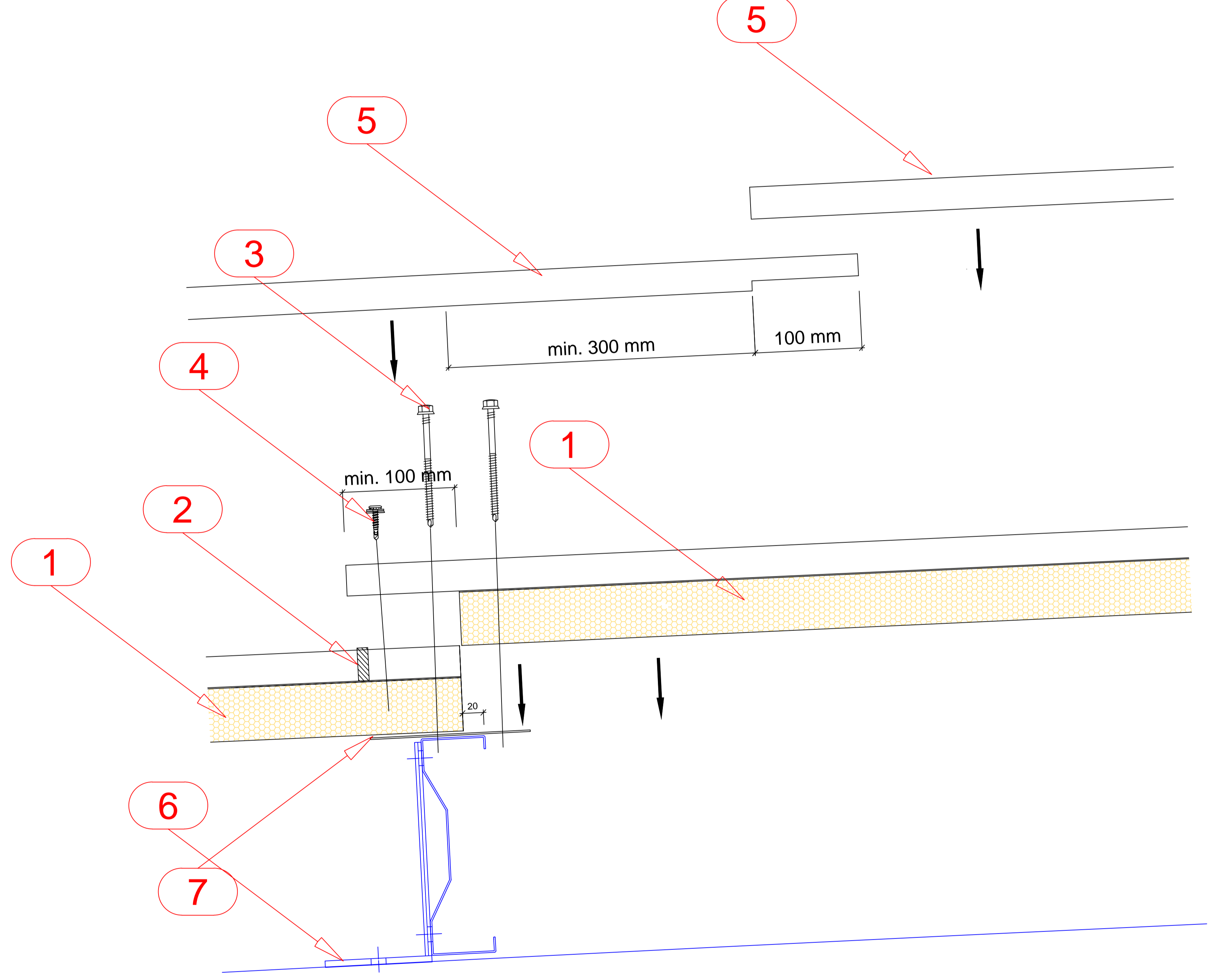
B NOKTA DETAYI ÖLÇEK 1/10
